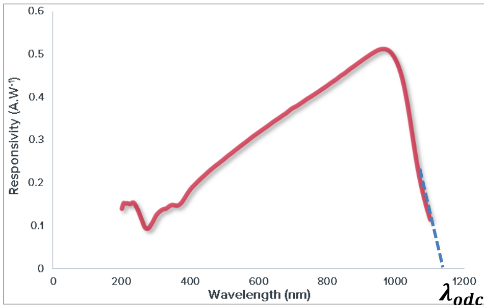
Czułość prądowa detektora Si
